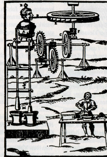
Abb. 5. Brancas Dampftrieb (1629). Ein Hüfischer B bläst einen Dampftrieb D gegen ein Schaufelrad E, das über ein Zahnradgetriebe F—L eine Pulverstampfe antreibt.
